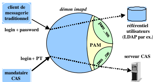
Figure 10 : Utilisation de pam_cas pour un serveur IMAP
