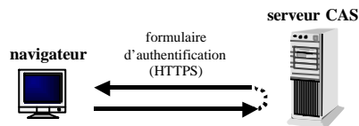
Figure 1 : Premier accès d'un navigateur au serveur CAS (sans TGC)
