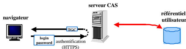
Figure 2 : Authentification d'un navigateur auprès du serveur CAS
